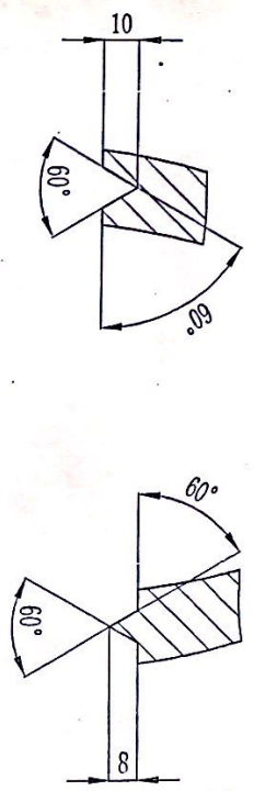
D-D M5:1
