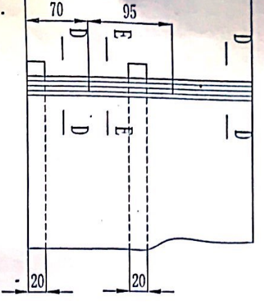
C向 M2:1
